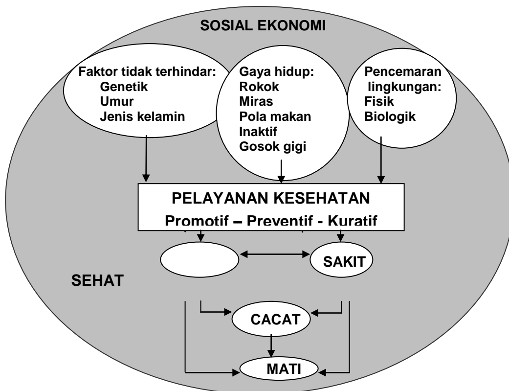
Gambar 1. Kerangka Konsep
